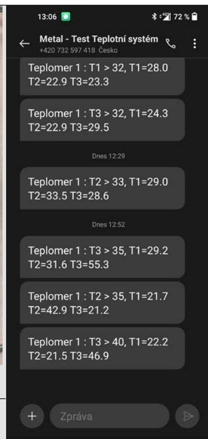
Vzor varovné zprávy o překročení teploty baterie
