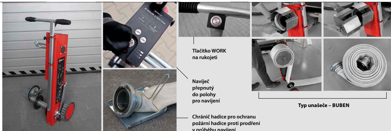
Složený navijec
